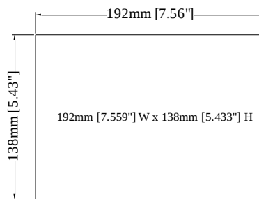
开孔尺寸图
