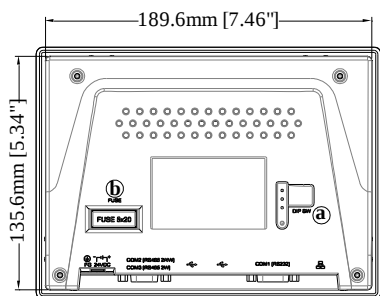
背视图
