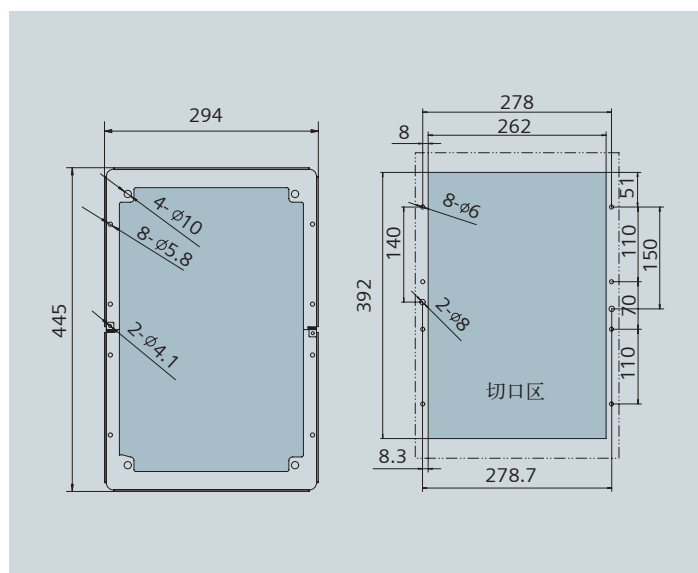
对应外形尺寸 D 变频器的穿墙式安装组件
