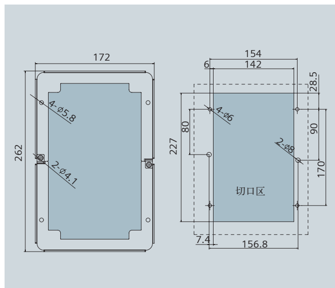
对应外形尺寸 A 变频器的穿墙式安装组件
