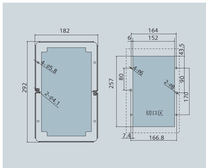
对应外形尺寸 B 变频器的穿墙式安装组件
