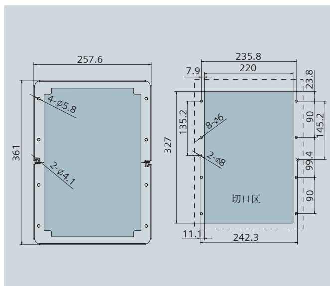
对应外形尺寸 C 变频器的穿墙式安装组件
