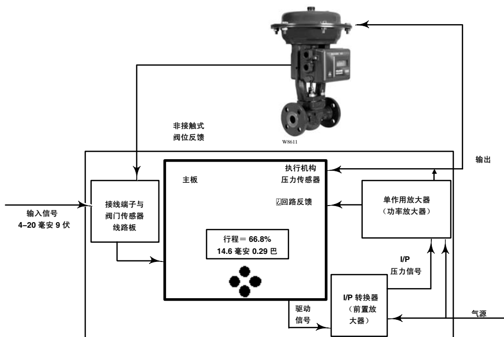
图 3. 模块图
