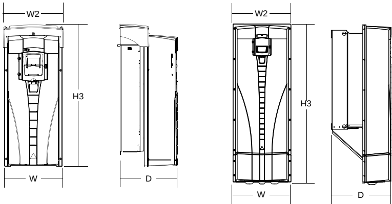
ACS550-01-290A-4, IP54 ( 不用于 UL 类型 12 ), 外形尺寸 R6
