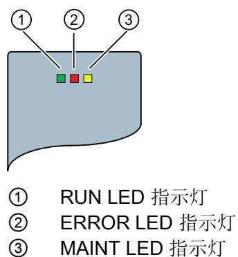
图 5-1 PS 60W 120/230V AC/DC 模块上的 LED 指示灯
