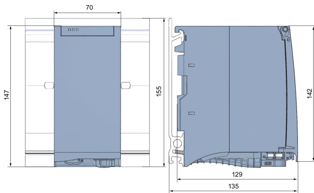
图 A-1 PS 60W 120/230V AC/DC 模块的尺寸图
