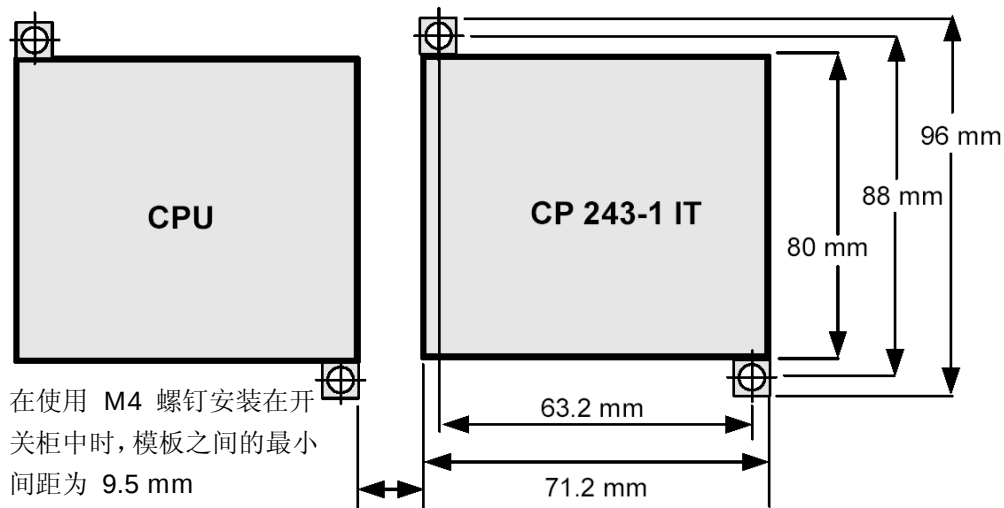
图 6 在控制面板中的安装尺寸
