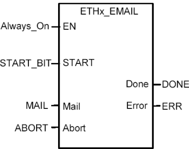
图 12 调用 ETHx_EMAIL 子程序
