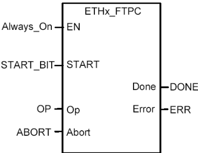
图 13 调用 ETHx_FTPC 子程序
