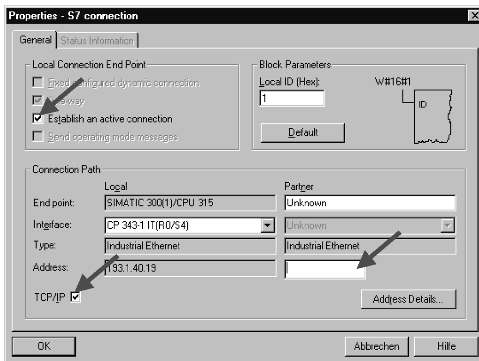
图 8. “S7 连接属性”对话框
