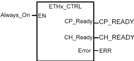
图 9. 调用 ETHx_CTRL 子程序
