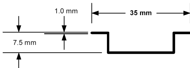
图 7 在 DIN 导轨中的安装尺寸
