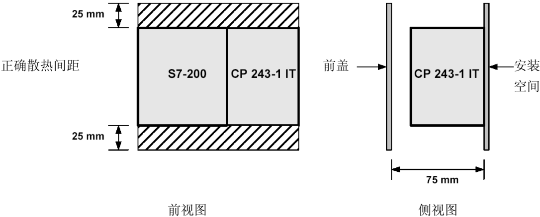
图 5. 安装空间要求
