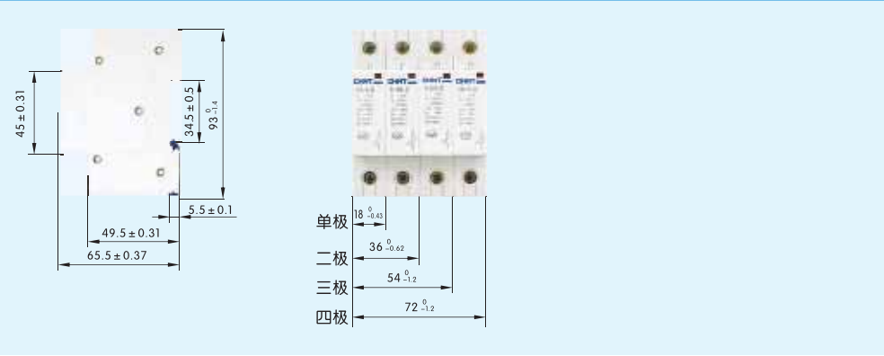
图4 NU6-II /F(100kA)带远程信号输出接点电涌保护器外形及安装尺寸
