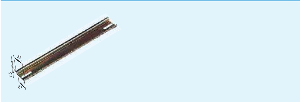
图6 TH35-7.5型安装导轨尺寸
