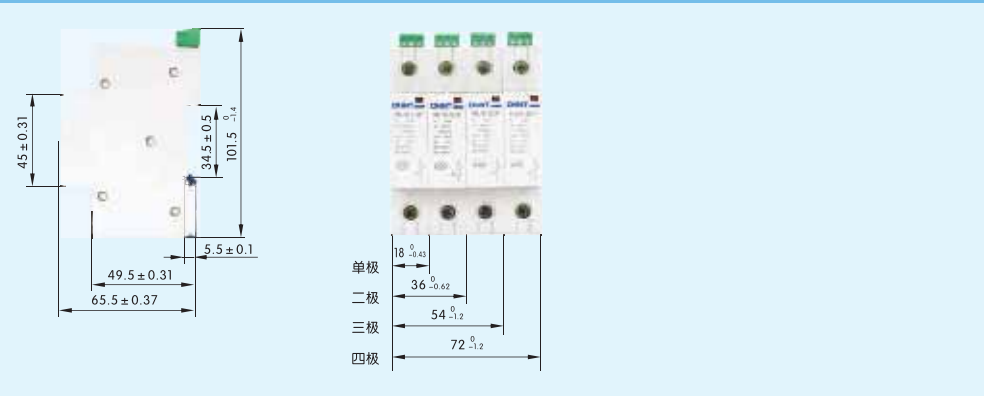
图2 NU6-II /F(40、60kA)带远程信号输出接点电涌保护器外形及安装尺寸
