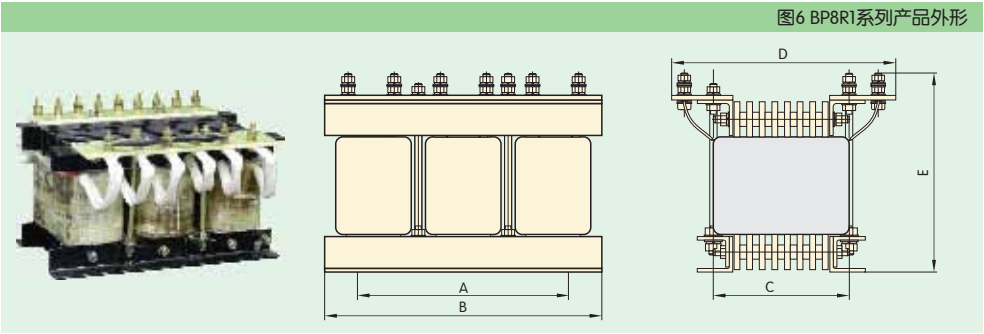
BP8R1系列产品外形和安装尺寸。
