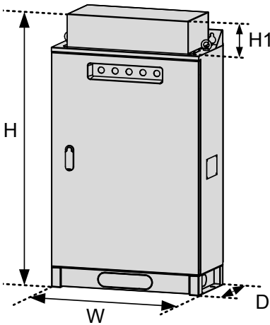
图 2-4 NICE-CB1 控制柜外观尺寸图
