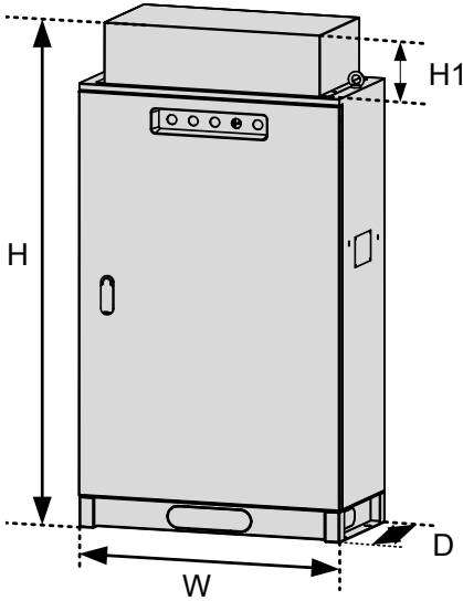
图 2-5 NICE-CE1 控制柜外观尺寸图
