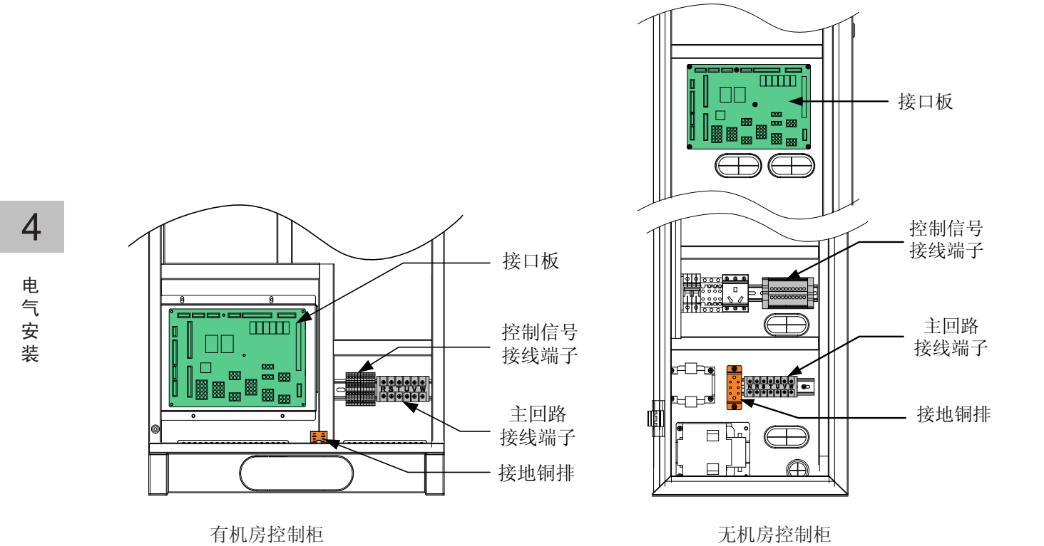
图 4-1 控制柜内部对外接口位置图
