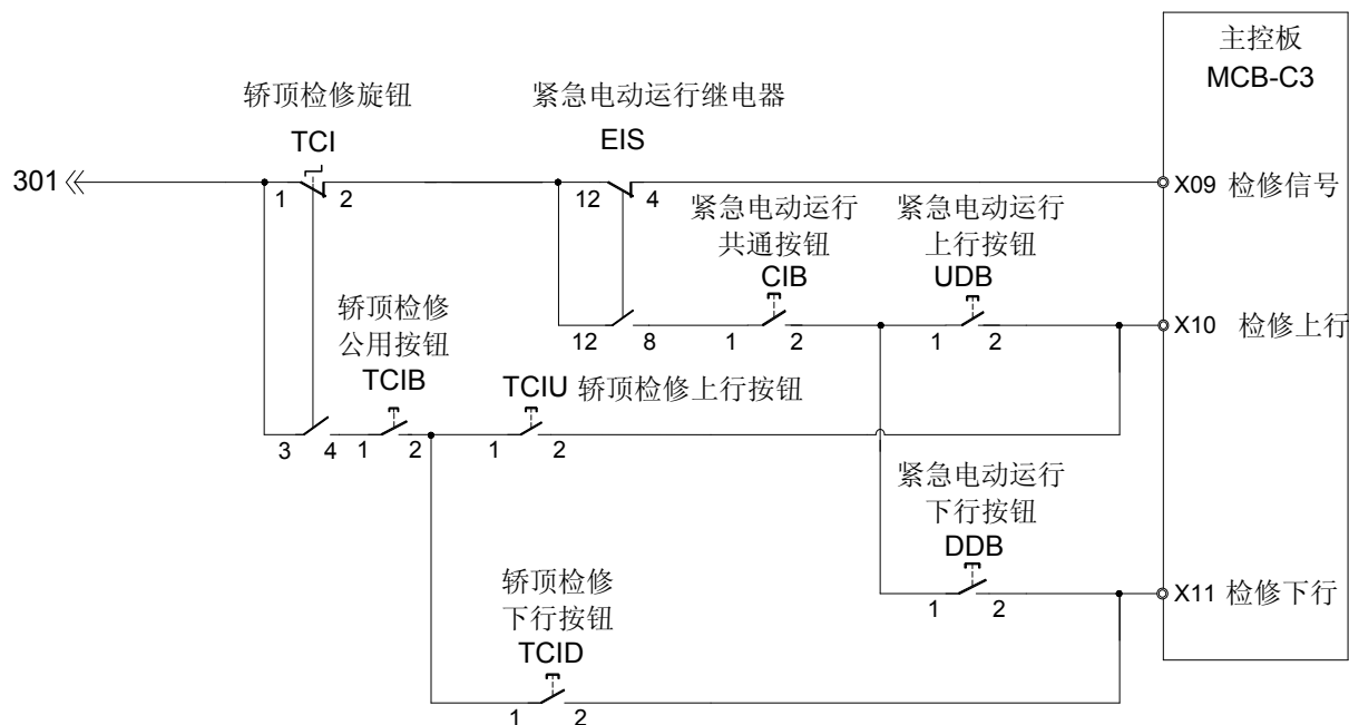
图 4-11 检修回路原理图
