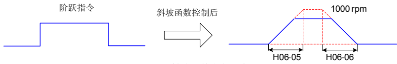
图 4-9 斜坡函数定义示意图
