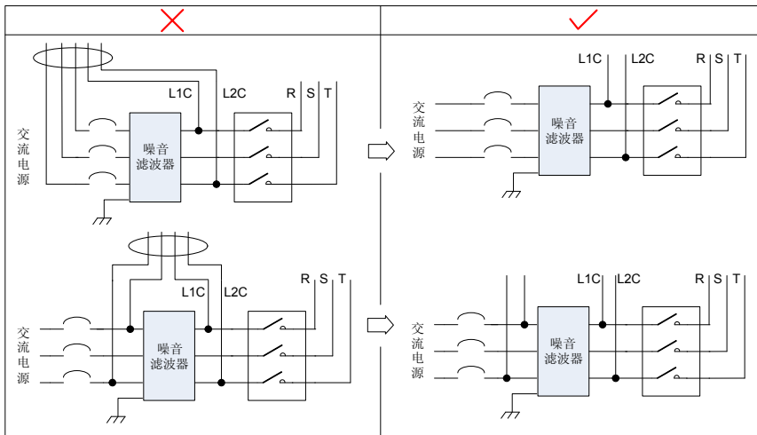
图 3-22 噪音滤波器输入与输出配线分离走线示意图
