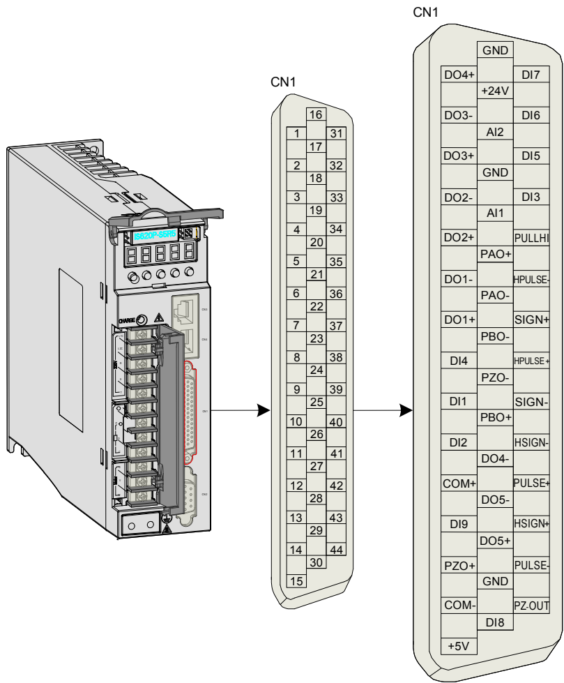
图 3-9 驱动器控制回路端子连接器引脚分布图
