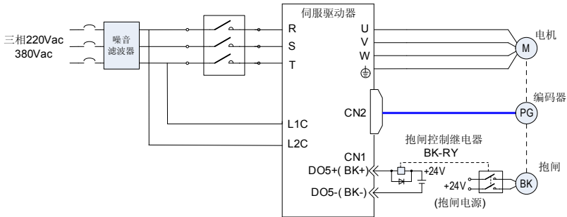
图 3-12 抱闸配线图
