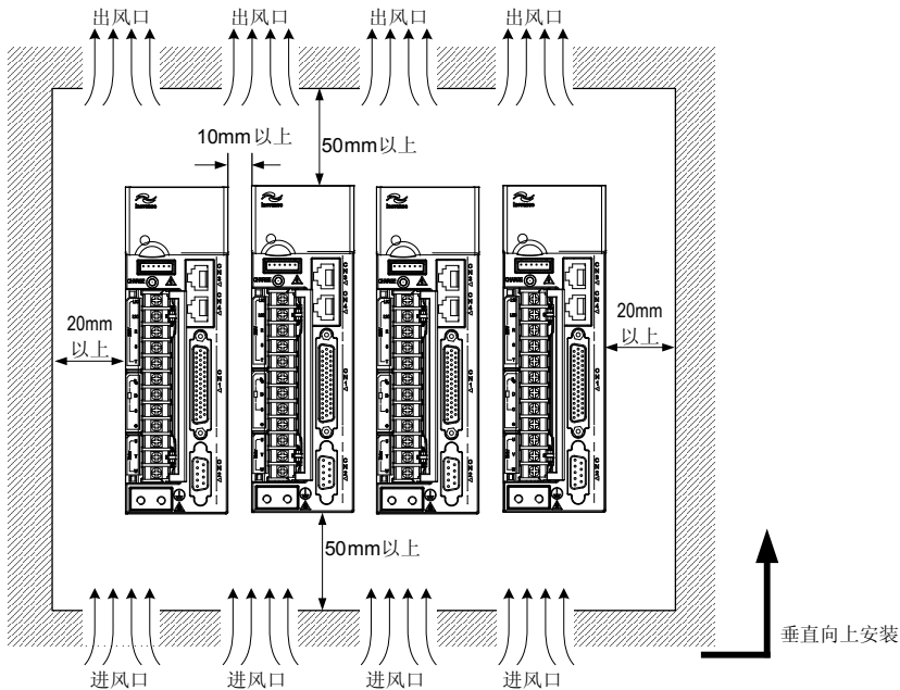
图 2-1 伺服驱动器安装示意图
