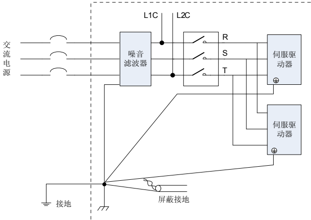
图 3-25 噪音滤波器地线处理示意图
