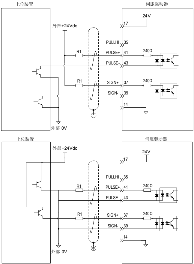
方案二：使用外接电阻
