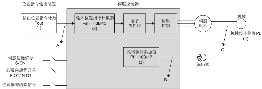
图 9-1 定位控制原理框图
