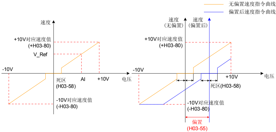
图 4-7 无偏置 AI2 示意图
