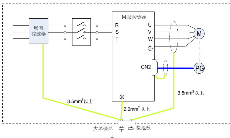
图 3-21 抗干扰配线实例
