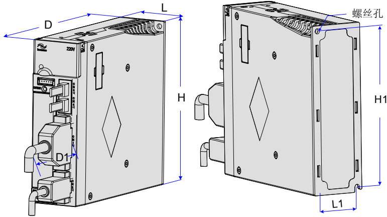
图 2-2 驱动器尺寸图
