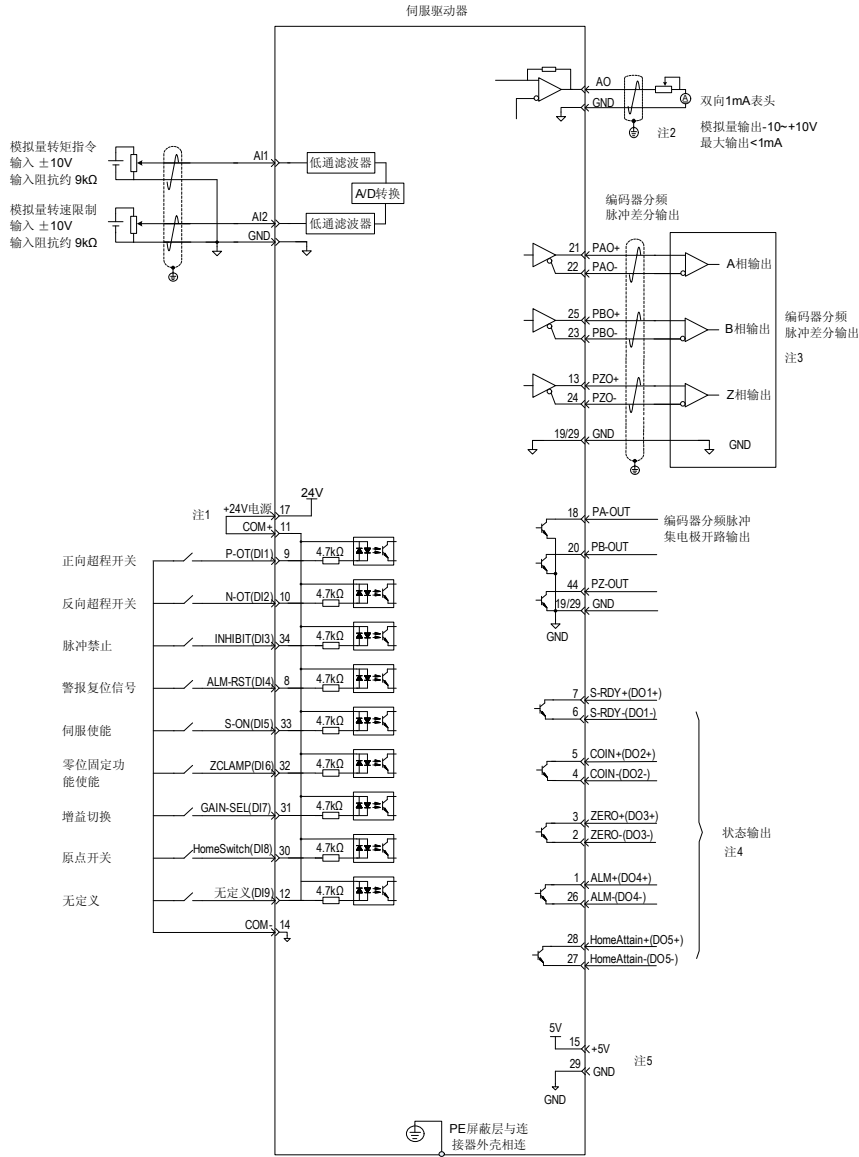
图 4-13 转矩模式配线图
