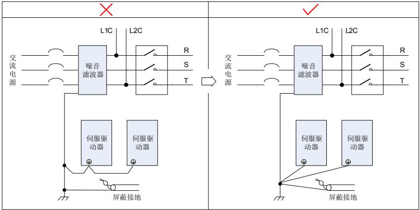
图 3-24 单点接地示意图
