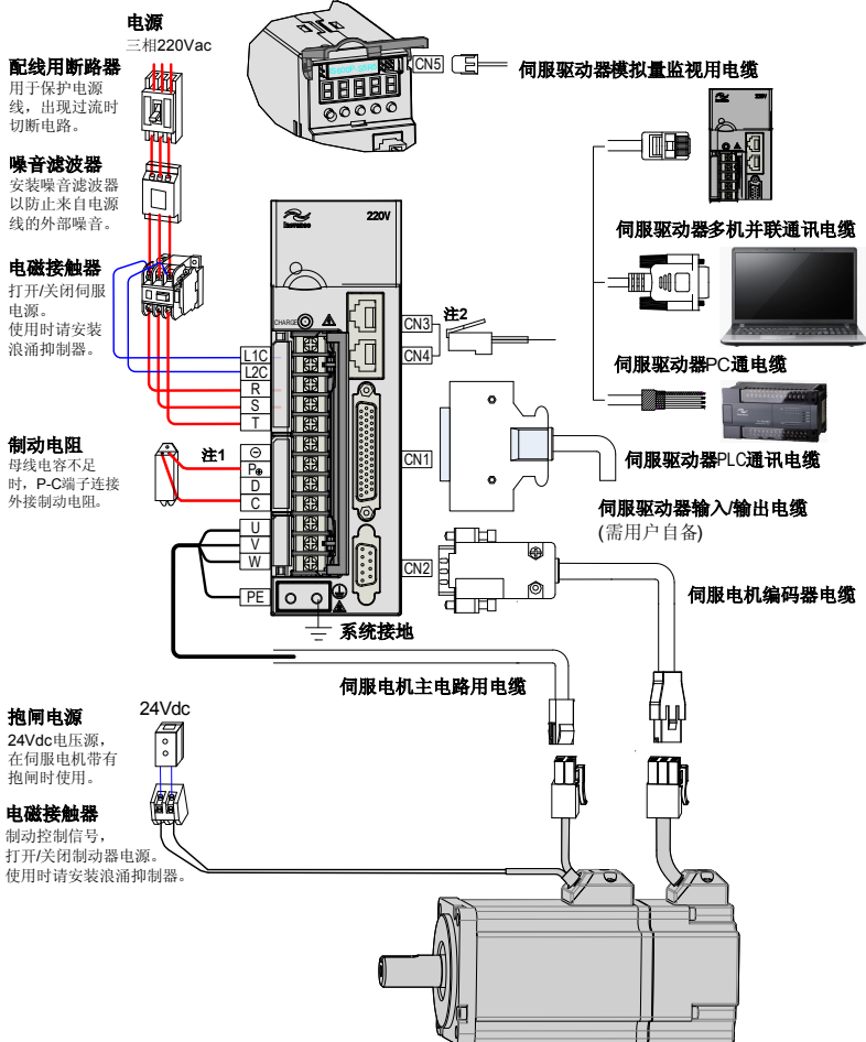
图 1-2 三相 220V 系统配线图举例
