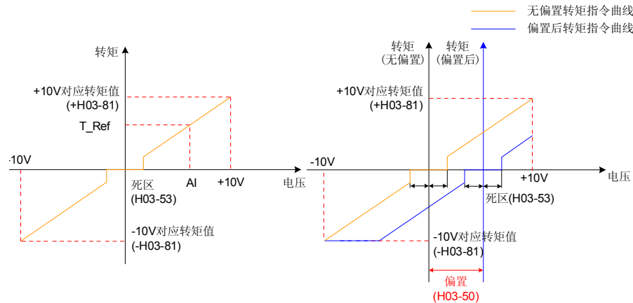
图 4-14 无偏置 AI1 示意图
