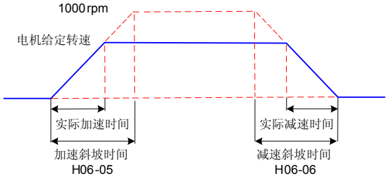
图 4-10 加减速时间示意图
