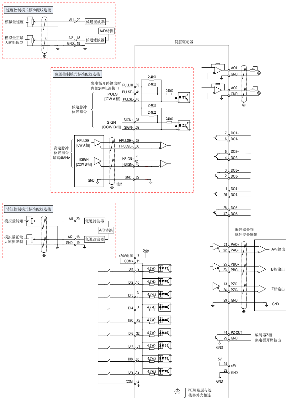
图 3-10 三种控制模式配线图举例
