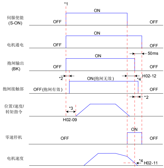
图 3-14 电机旋转时抱闸时序图
