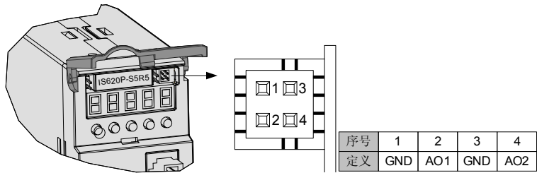
图 3-20 模拟量监视信号连接器端子
