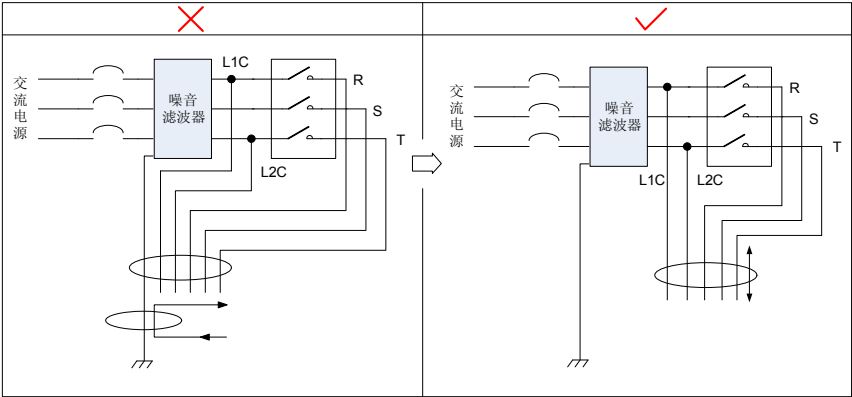
图 3-23 噪音滤波器地线与输出配线分离走线示意图
