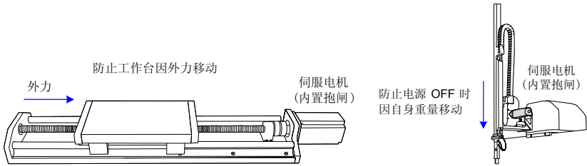
图 3-11 抱闸应用示意图
