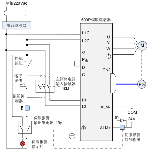
图 3-5 单相 220V 主电路配线
