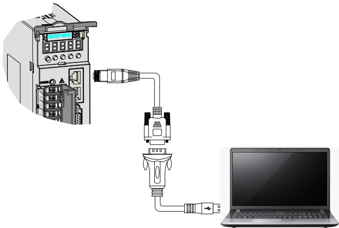
图 3-17 通讯串口转 USB 示意图
