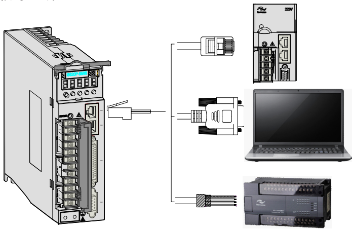
图 3-15 通信配线示意图
