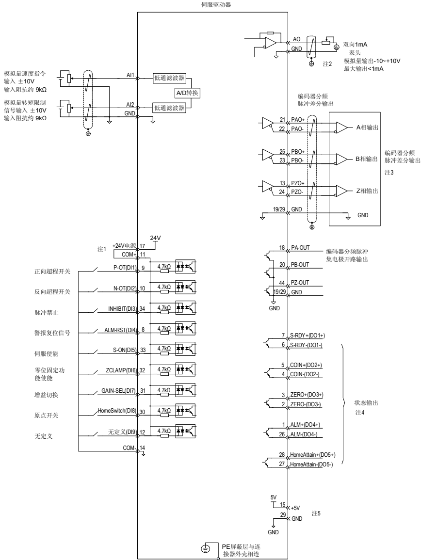
图 4-6 速度模式配线图
