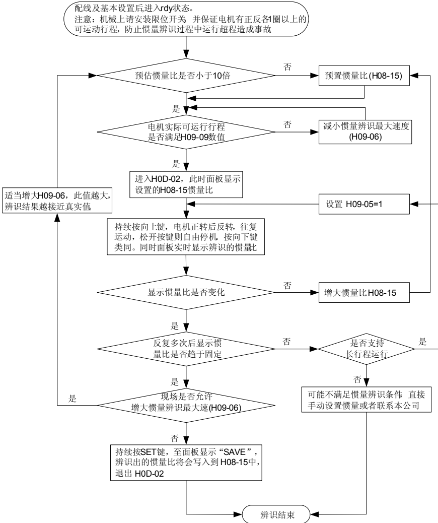
图 4-17 惯量辨识调试流程图
