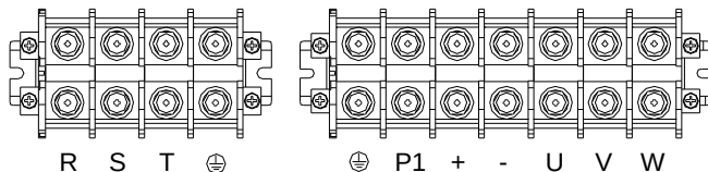
160kW 及以上标准品主回路端子
