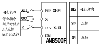
图 7- 5 3 线制顺序控制模式 1
