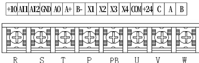
图 1-2 控制回路端子和主回路端子配置
