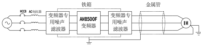
图 3-9 射频干扰措施
