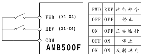
图 7- 4 2 线制顺序控制 2
