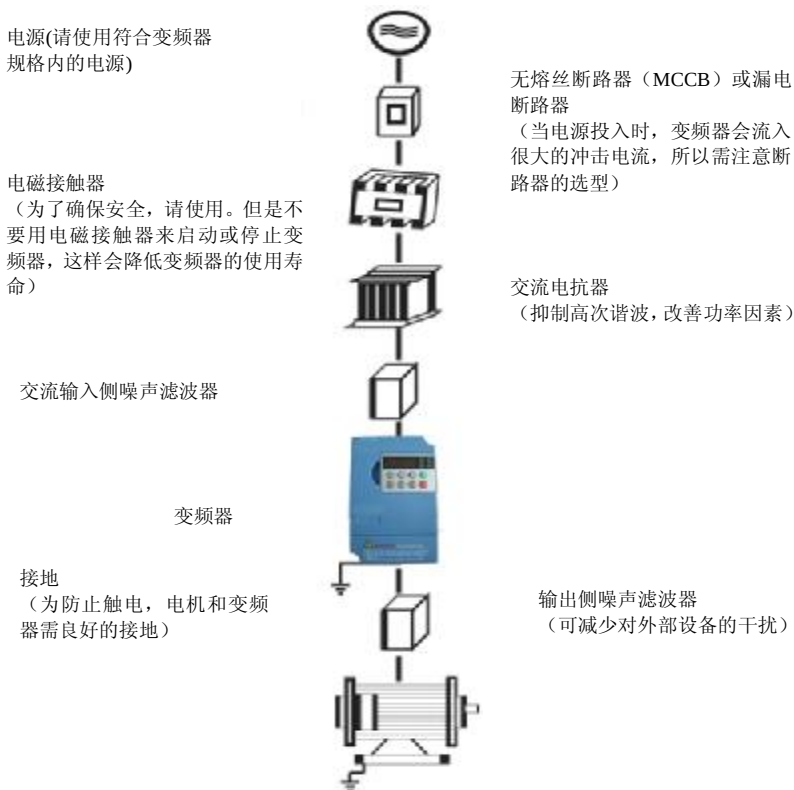
图 3-1 与外围设备的连接图
