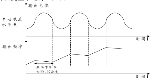
图 7-21 过流失速功能
