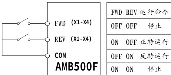
图 7- 3 2 线制顺序控制 1
