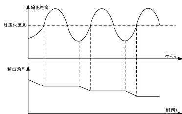
图 7-20 过压失速功能
