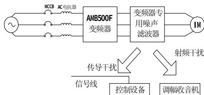
图 3-7 输出侧噪声滤波器的安装
