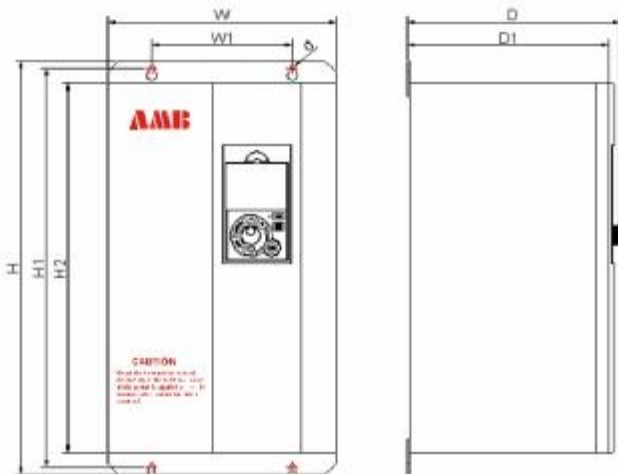
160KW 及以上规格外形尺寸
