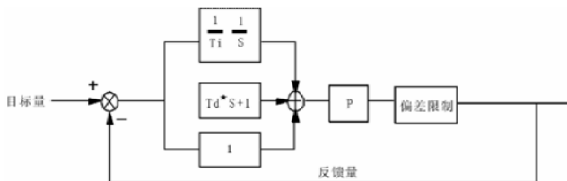
图 7-18 过程 PID 原理框图
