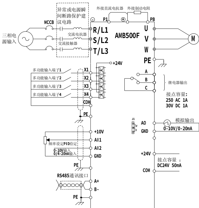
图 3-2-2 AMB500F (11-400KW) 变频器连接图
