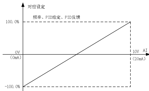
图 7- 7 模拟给定与设定量的对应关系
