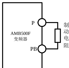
图 3-11 制动电阻的安装
