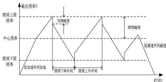
图 7-15 摆频运行示意图
