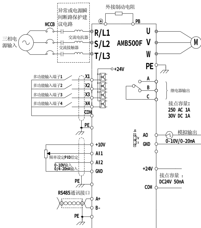
图 3-2-1 AMB500F (0.4-7.5KW) 变频器连接图
