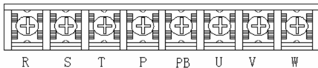
三相 220V/380V(0.75-7.5KW)主回路端子
