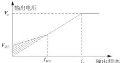
图 7-12 手动转矩提升示意图
