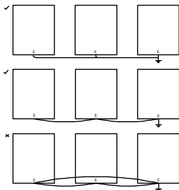
图 3-10 接地线连接方法
