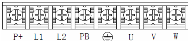
单相 220V (0.4-1.5KW)主回路端子
