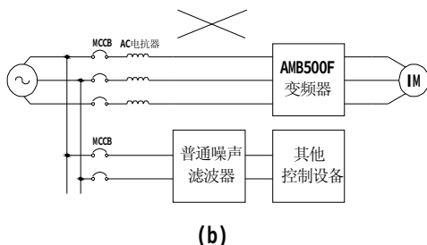
图 3-6 噪声滤波器的错误设置
