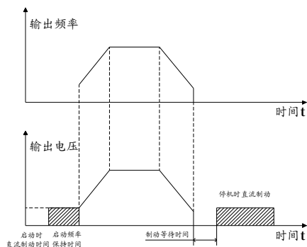
图 7-9 直流制动示意图
