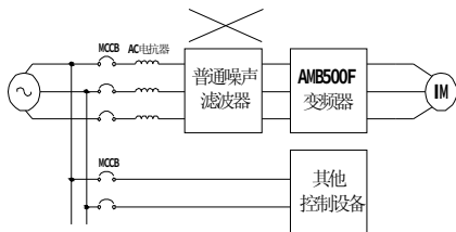
图 3-5 噪声滤波器的正确设置
