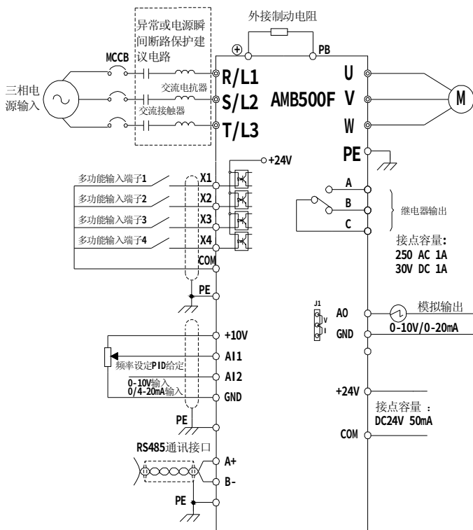
图 3-13 控制回路端子连接图
