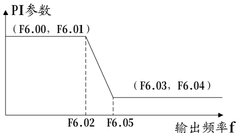
图 7-13 PI 参数示意图
