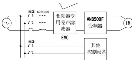
图 3-5 噪声滤波器的正确设置
