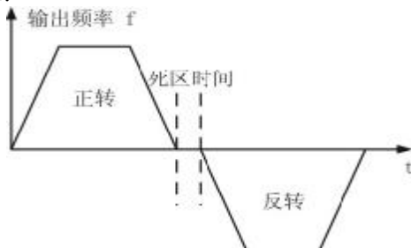
图 7-10 正反转死区时间示意图
