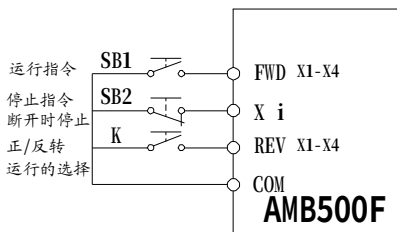
图 7-6 3 线制顺序控制模式 2
