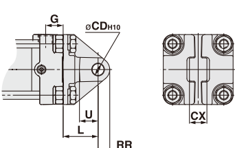
单耳环型
