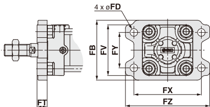
法兰型
