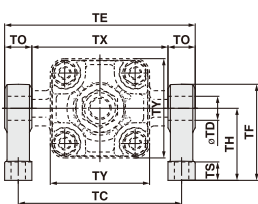
耳轴脚座
