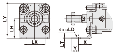
脚座型
