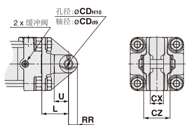
双耳环型
